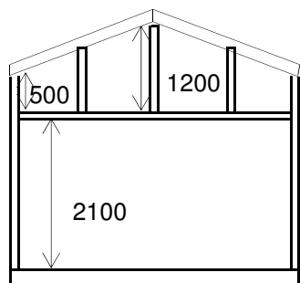
SEKTION A
